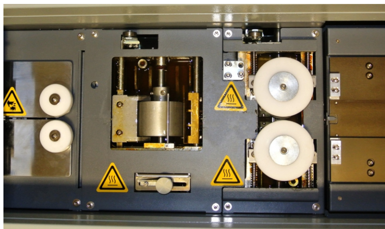
Два разных клеевых резервуара для более сильного склеивания
